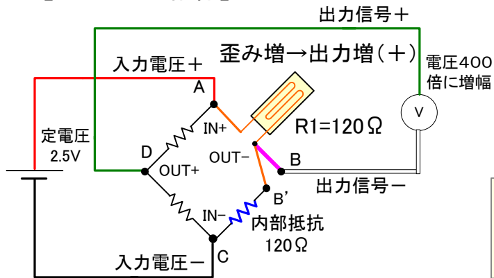
【1ゲージの結線】
