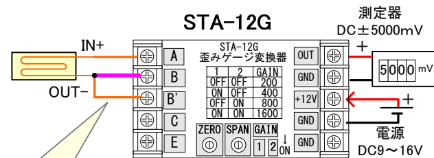
【実際の結線：1ゲージ：120Ω 3線式】
