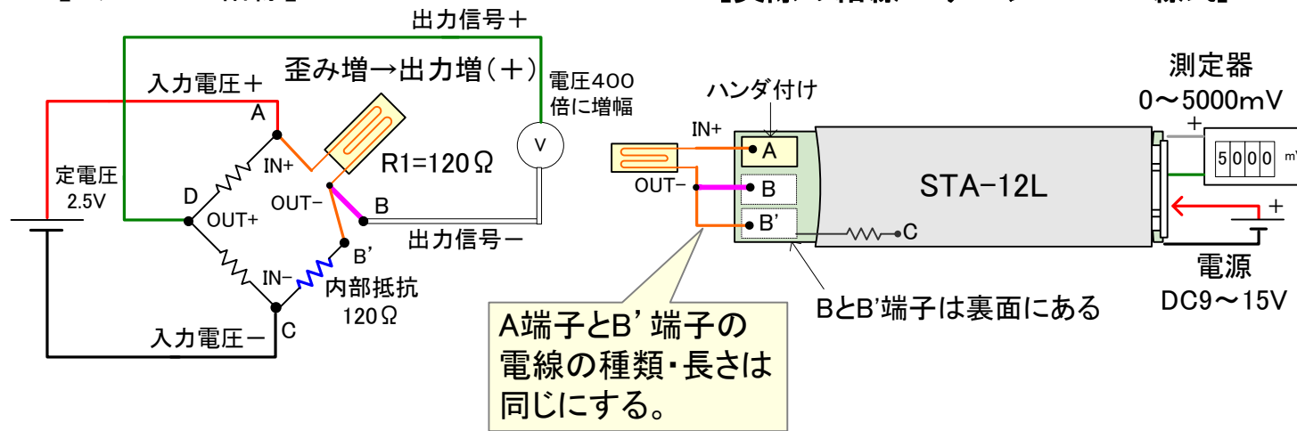
【1ゲージの結線】
