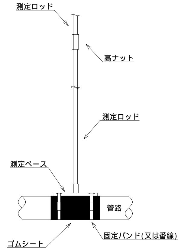
沈下棒組立図
